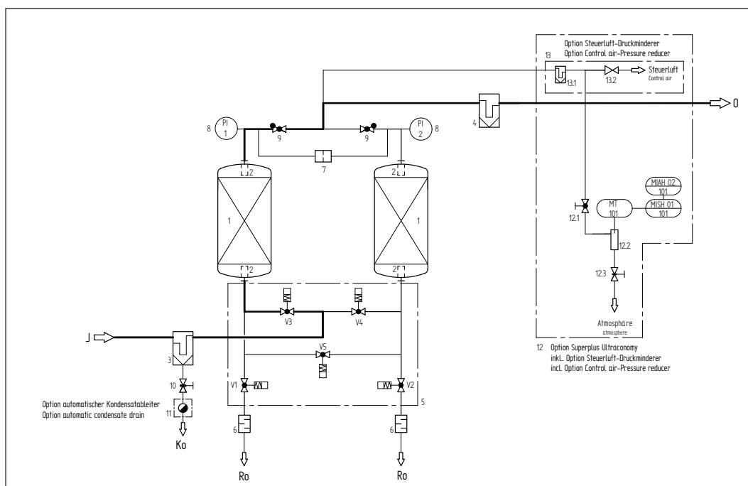
Hochdruck-Adsorptionstrockner HLP 0260-1200
