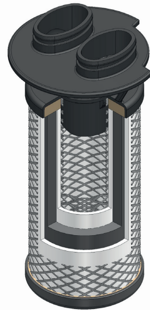
Querschnitt durch den Tiefenfilter A
