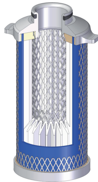
Querschnitt durch den Tiefenfilter
