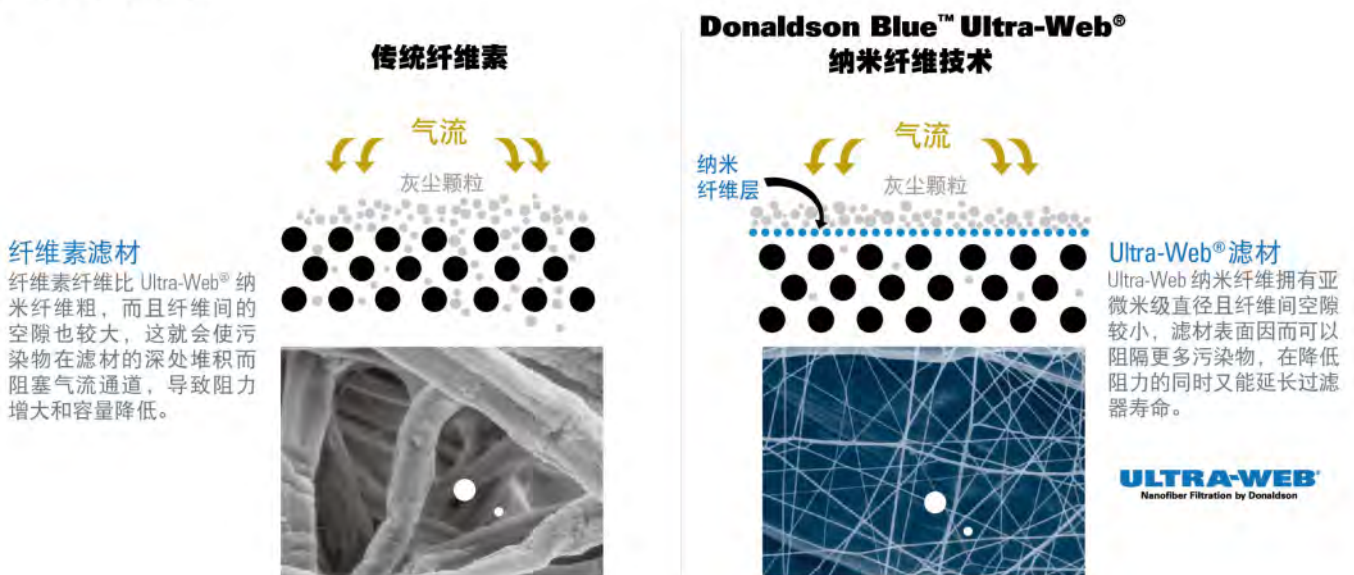
放大后的滤材俯视图（放大倍数相同） 色圆点分别代表直径为 2 \mu 和 5 \mu 的颗粒。
